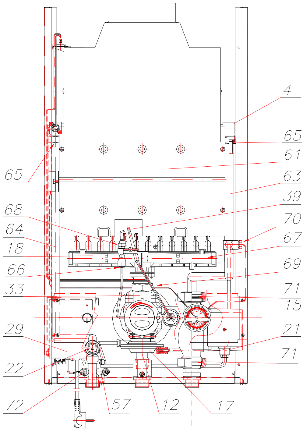
Rys.6. Podstawowe elementy kotła typ GCO-20-00
