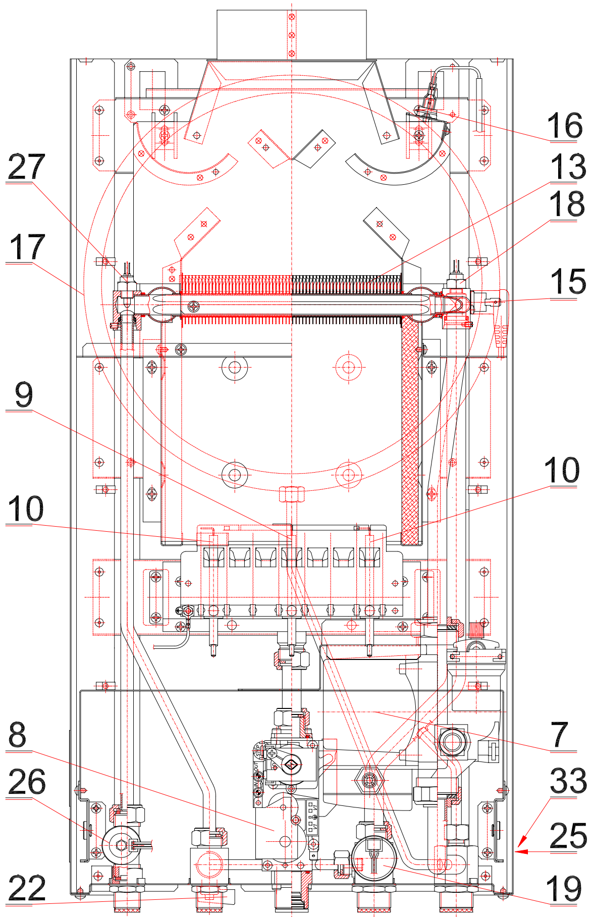
Podstawowe elementy kotła typ GCO-DP-14-00
