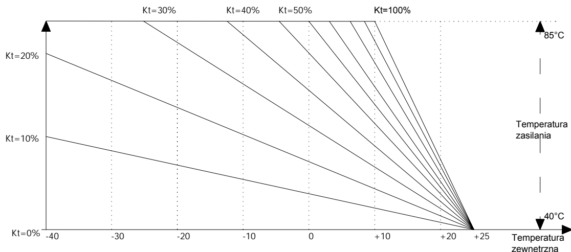
Rys. 2.4.1.1.1. Krzywa grzewcza
