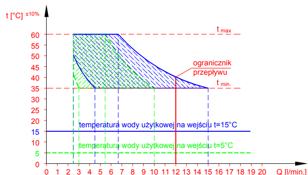
Rys. 2.4.2.1. Wykres temperatury wody użytkowej na wyjściu z kotła w zależności od wielkości przepływu wody
