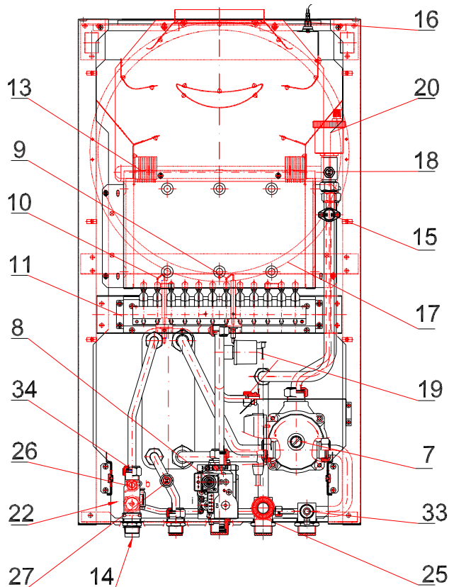
Rys. 2.2.1.1 Rozłożenie elementów w kotle
