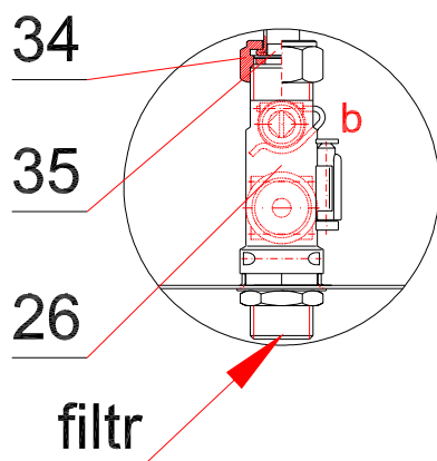
Rys. 6.1.5.1. Usytuowanie ogranicznika przepływu w kotle
