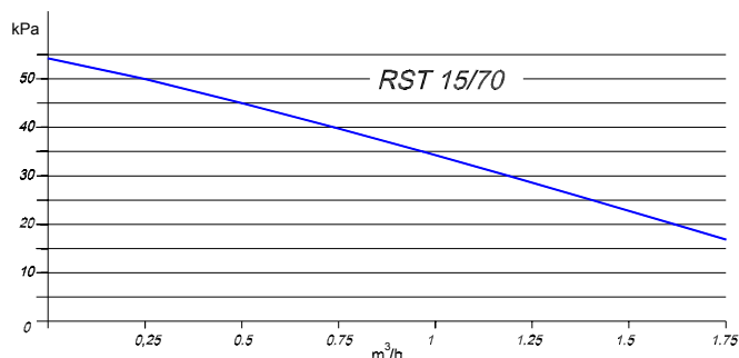
Rys. 6.2.11.1 Charakterystyka pompy
