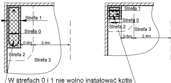
Rys. 3.1.2.1. Miejsce instalowania kotła w pomieszczeniu wyposażonym w wannę lub basen natryskowy zgodnie z wymaganiami zawartymi w PN-IEC 60364-7-701.
