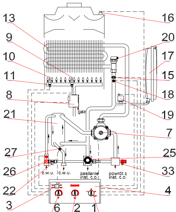
Rys. 2.2.1.2 Schemat ideowy działania kotła
